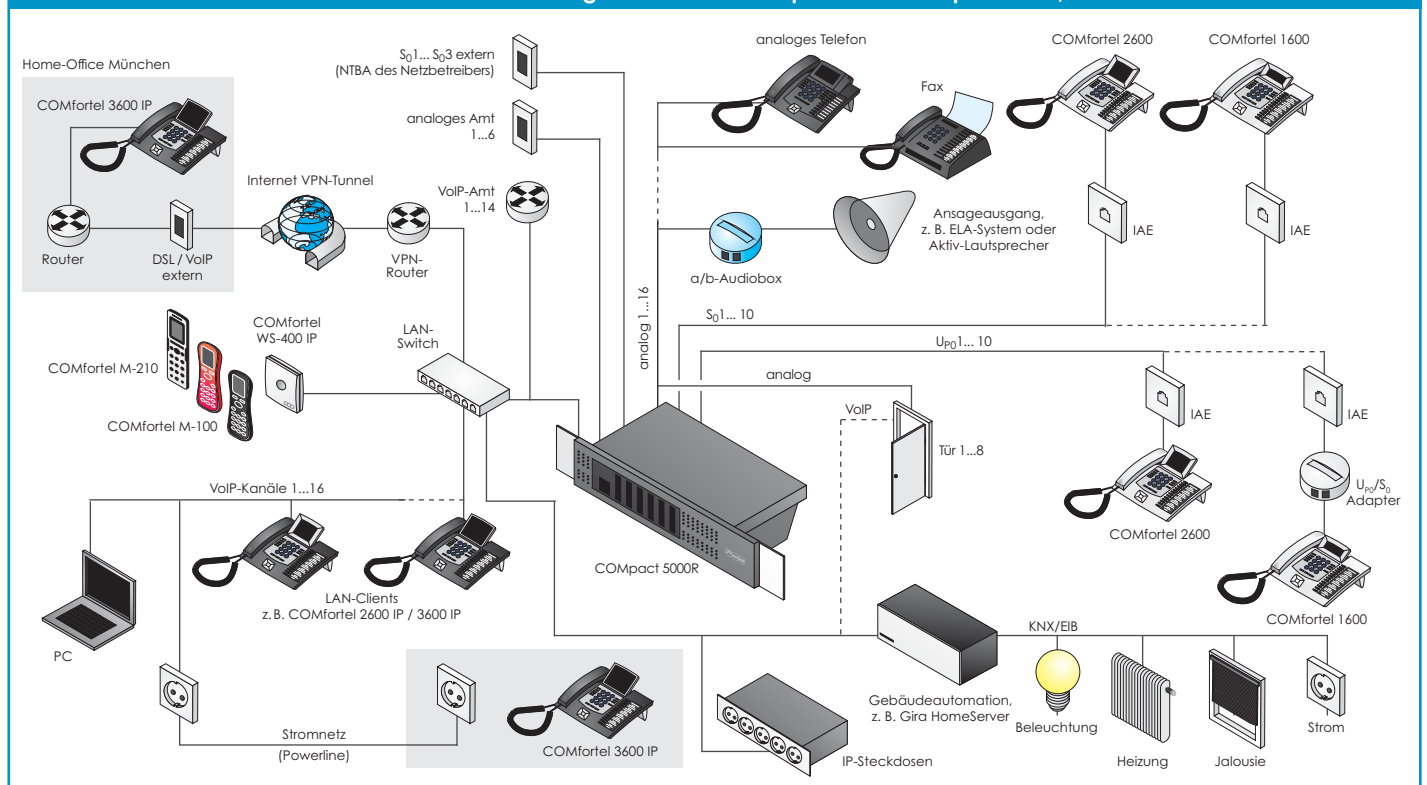
Ausbau- und Anschlussmöglichkeiten am Beispiel einer COMcompact 5000/5000R
